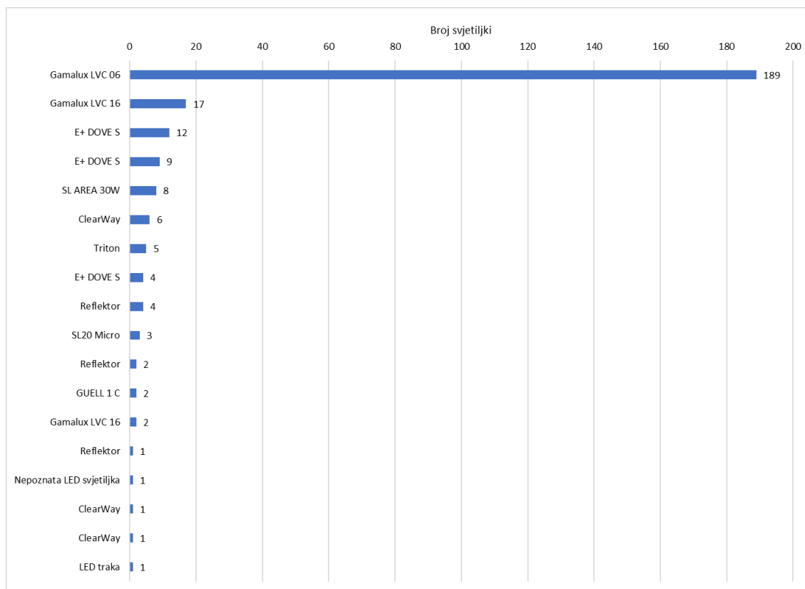
Slika 8. Struktura sustava javne rasvjete prema tipu svjetiljke
